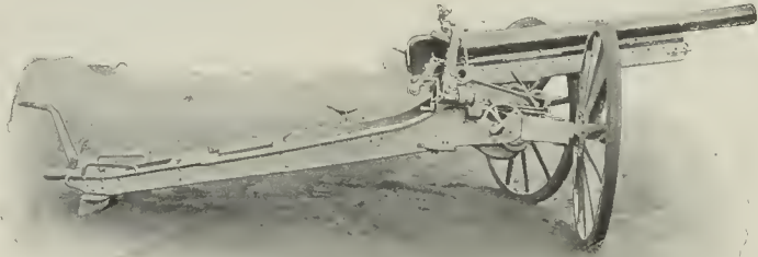
Cañón Krupp de 45 centímetros en su cureña de campaña
